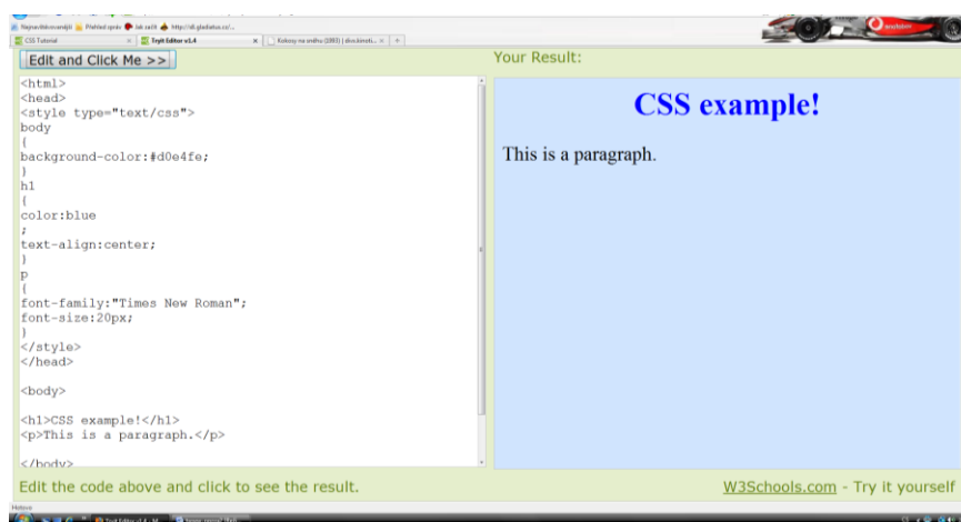
Obr. 9 CSS Zkoušečka
