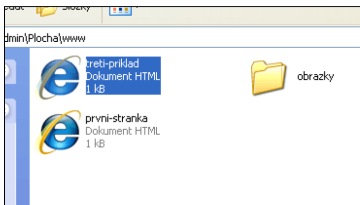
Obr. 5 Relativní odkazování
